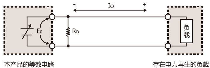
本产品的等效电路
